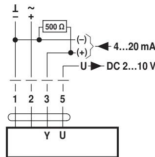
Aansturing met 4...20 mA via externe weerstand
