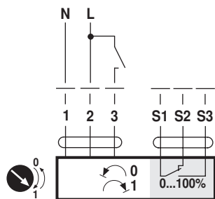
AC 230 V, tout-ou-rien
