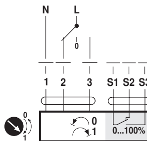
AC 230 V, 3 points
