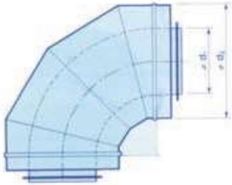
Dempende bochten met 50 mm isolatie Coudes d'insonorisation - isolation 50 mm
